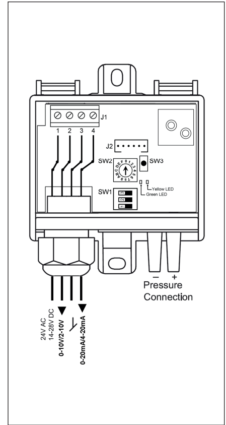
Fig. 3 - Wiring diagram
