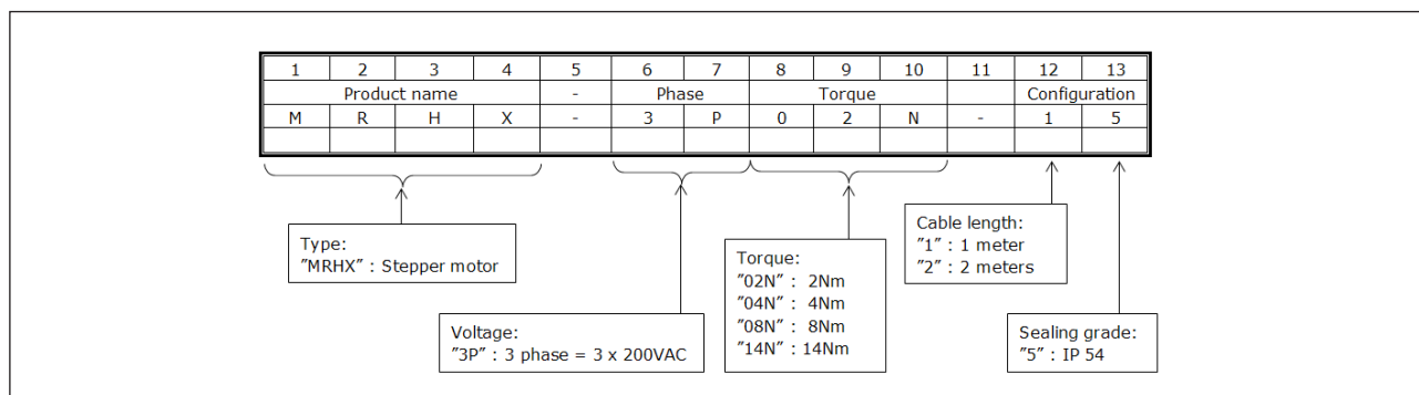
Figur 10.6.2 - Steppermotor; produkt ID
