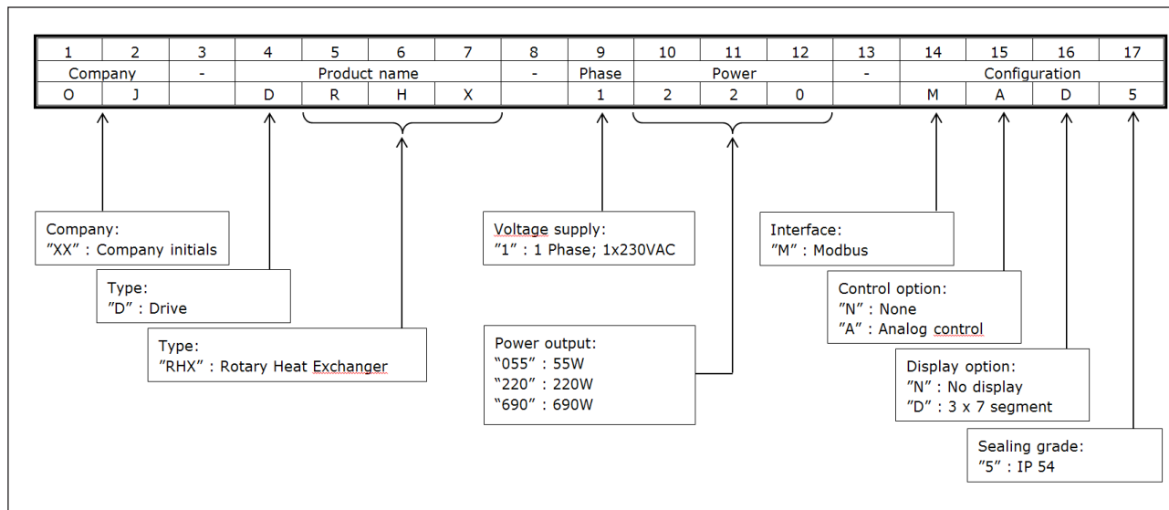
Figur 10.6.2 - Steppermotor; produkt ID
