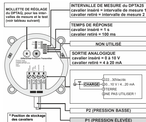
Fig. 6. Détails de câblage
