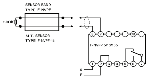
Tilslutningsdiagram
